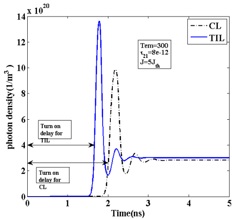
شکل ۳. چگالی فوتون بر حسب زمان به ازای یک چگالی جریان ثابت برای دو حالت CL و TIL.
