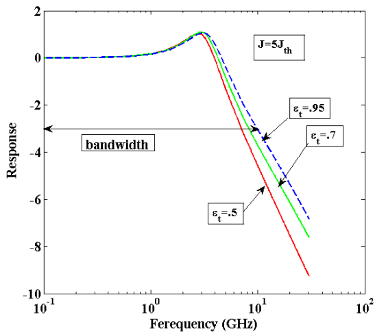
شکل ۵. تابع پاسخ مدولاسیون را به ازای \epsilon_f های مختلف.
