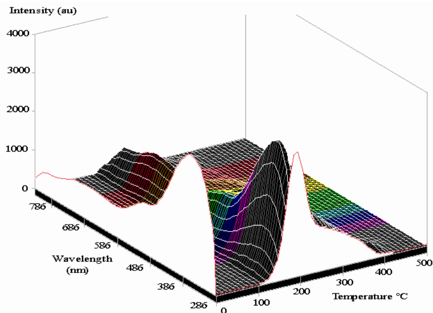
شکل ۷. طیف تابش نمونه \text{LiF}(\text{Cu}^{2+}) پرتودهی با 700 \text{ Gy} گری چشمه بتا
