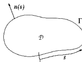
شکل ۳. تصویر یک بیلارد D بعدی که یک مرز D-1 بعدی آن را محصور کرده است.
