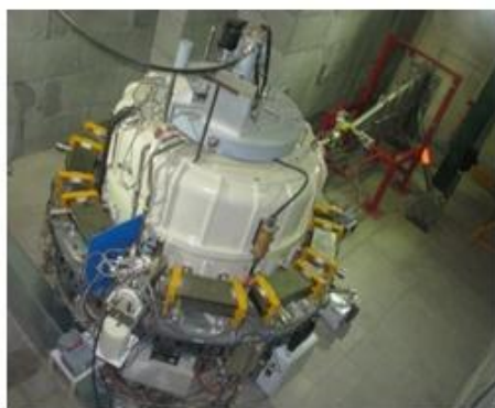
شکل ۶. شتاب‌دهنده پر قدرت صنعتی الکترون ساخته شده و بخشی از اتاق کنترل این شتاب‌دهنده.
