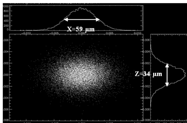
شکل ۲. اندازه و توزیع باریکه فوتونی در مکان نمونه با استفاده از Shadow (تعداد پرتوها 25000 ).
