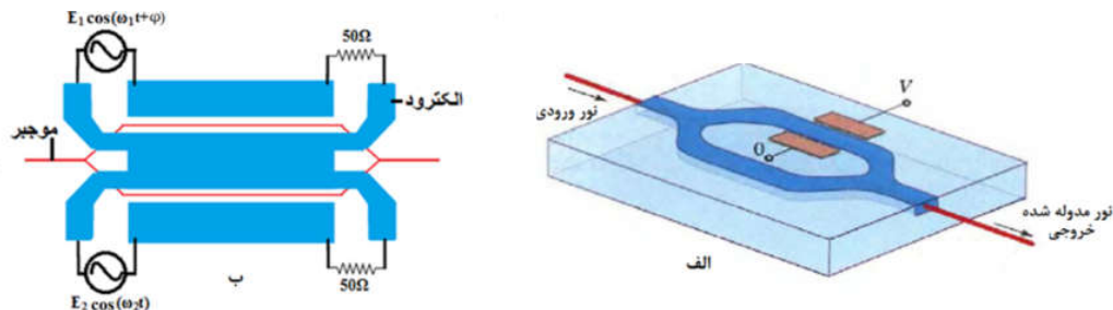
شکل ۱. (رنگی در نسخه الکترونیکی) (الف) طرحواره یک مدوله‌کننده ماخ-زندر با تحریک یکی از شاخه‌های موجبر (ب) طرح‌واره مدوله‌کننده هتروداين ساخته شده.
