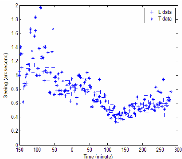
شکل ۳. نمودار \epsilon_l و \epsilon_t را در طول یک شب نشان می‌دهد. محور افقی زمان بر حسب دقیقه است و زمان ۰ نیمه شب را نشان می‌دهد.
