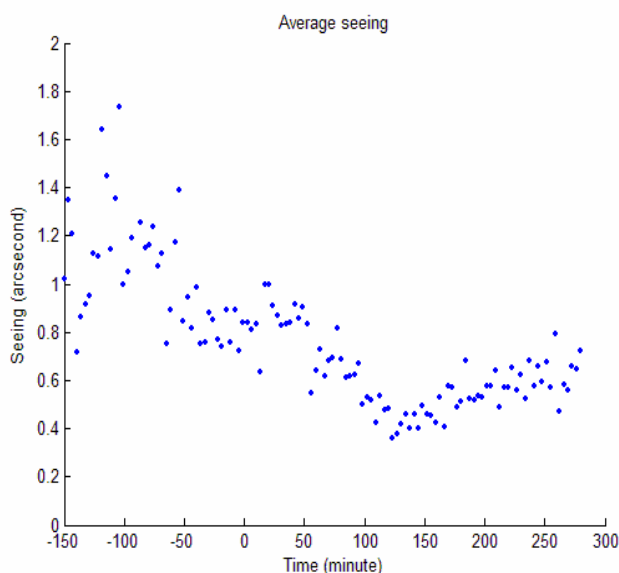
شکل ۴. نمودار \bar{\epsilon} نظیر شکل ۳ را در طول یک شب نشان می‌دهد.
