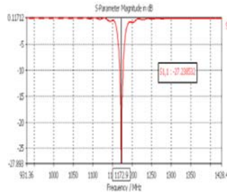
شکل ۲. نتایج شبیه‌سازی و تجربی توان برگشتی از درگاه مرکزی.
