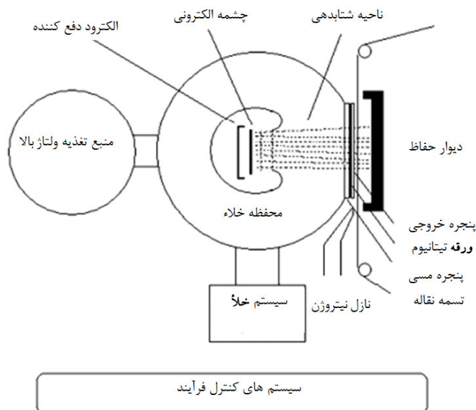
شکل ۱. طرح واره‌ای از شتاب دهنده پرتوهای الکترون [۱].
