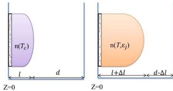
شکل ۴. (رنگی در نسخه الکترونیکی) نمادینی از OPD ناشی از انبساط حرارتی. در این شکل، مستطیل‌های نقطه چین سینک حرارت (چاه حرارت) را نشان می‌دهند.
