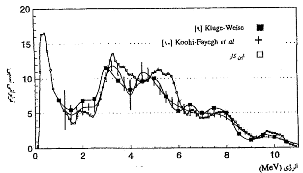
شکل ۴ مقایسه طیف محاسباتی چشمه \alpha -Be با نتایج تجربی.
