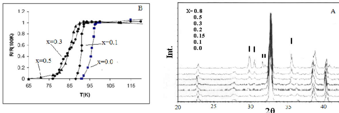
شکل ۱ (A). نمایه‌های XRD به ازای مقادیر متفاوت آرایش پتاسیم. (B) تغییرات دمای بحرانی ابر رسانایی به ازای آرایشهای مختلف [۷]. قله‌های مربوط به ناخالصی با نشانه‌هایی در بالا معین شده‌اند.
