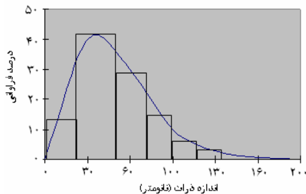
شکل ۲. توزیع اندازه ذرات شکل ۱.
