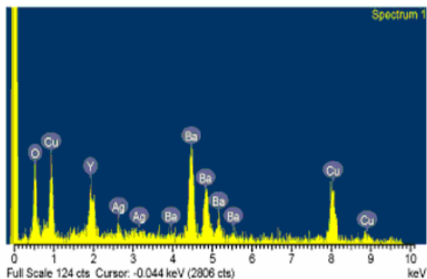
شکل ۳. طیف EDX نمونه ابرسانی YBCO با حضور Ag.
