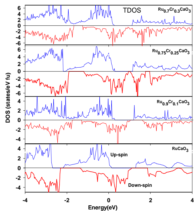
شکل ۲. چگالی حالات کل و برآورد انرژی شکافتگی تبدیلی برای Ru_{1-x}Cr_xCaO_3 .
