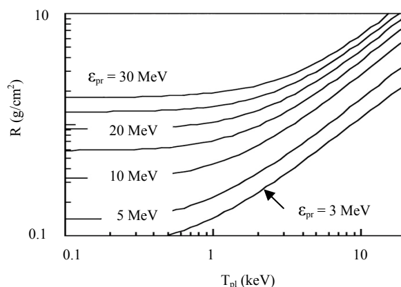
شکل ۲. نمودار برد پروتونی R بر حسب دمای پلاسما، T_{pl} ، برای پروتون‌های با انرژی اولیه \epsilon_{pr} در پلاسمای D-T با چگالی 400 \text{ g/cm}^3 [۱۱].
