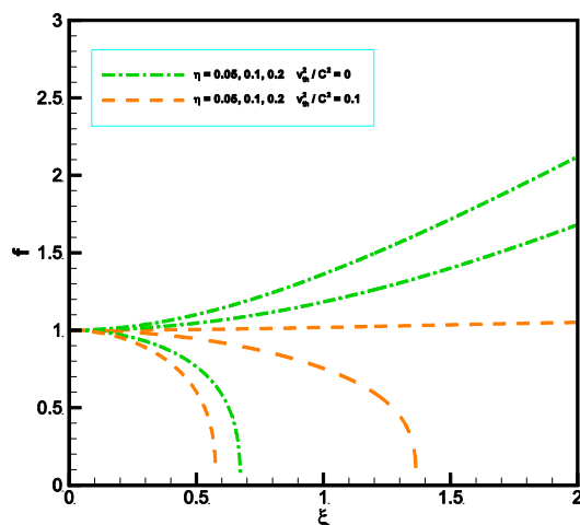
شکل ۱۲. تغییر پهنای لیزر برای مقادیر \eta = 0.05, 0.1 با فرض (\frac{v_{th}}{c})^2 = 0 و \eta = 0.05, 0.1, 0.2 .
