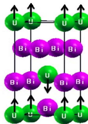
شکل ۱. ساختار مغناطیسی بلور پادفرومغناطیس UBi_2
