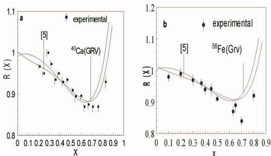
شکل ۲. در نمودار a و b نسبت R(x) = \frac{F_V^A}{F_V^D} که تابعی از x برای هسته‌های ^{40}\text{Ca} و ^{56}\text{Fe} است با در نظر گرفتن اثرات انرژی بستگی هسته‌ای محاسبه شده است و داده‌های تجربی از مرجع [۱۳] گرفته شده‌اند.
