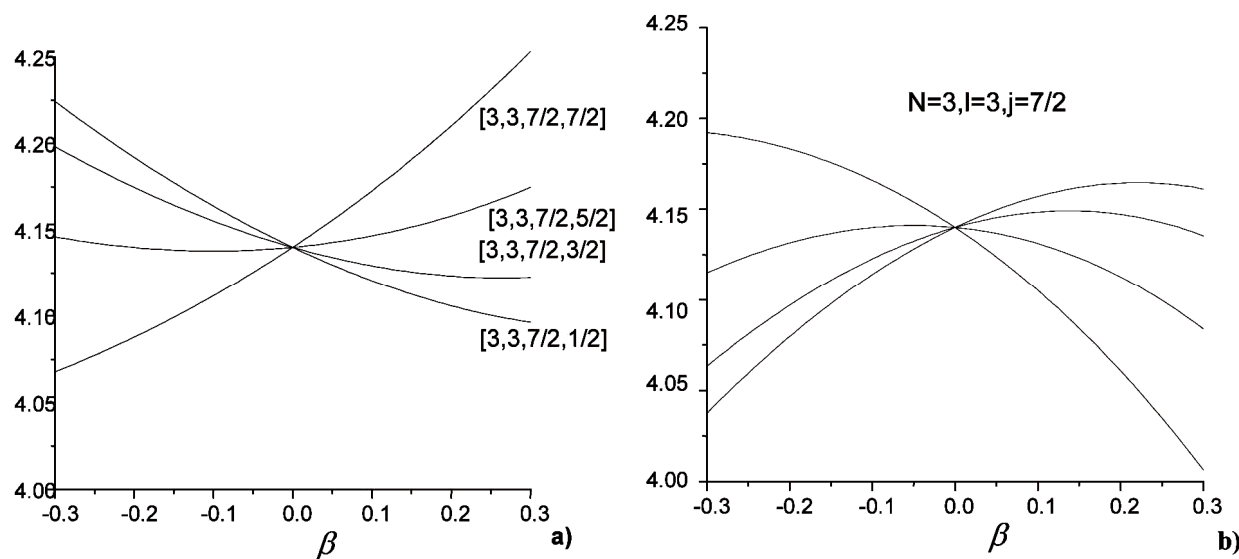
شکل ۶. ترازهای مختلف انرژی به واحد \hbar\omega_0 برحسب پارامتر تغییر شکل \beta (a) مدل نیلسون N=3, l=3, j=\frac{7}{2} و (b) مدل تغییر شکل یافته سه محوری N=3, l=3, j=\frac{7}{2} .
