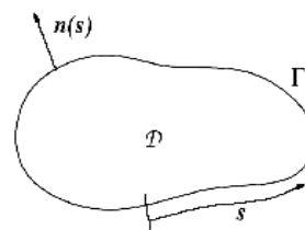
شکل ۳. تصویر یک بیلیارد D بعدی که یک مرز D-1 بعدی آن را محصور کرده است.
