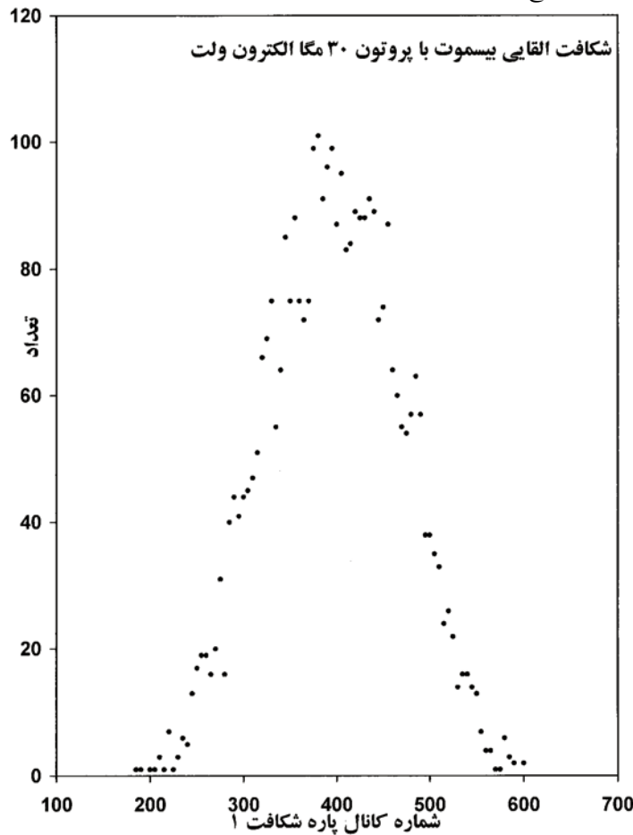
شکل ۲. توزیع یک پارامتری تعداد فرایند شکافت همفروود برحسب شماره کانال انرژی پاره شکافت ۱ در واکنش بیسموت با پروتونهای ۳۰ MeV. آشکارساز ۲ در زاویه ۹۰ درجه نسبت به راستای باریکه تابشی قرار گرفت.
