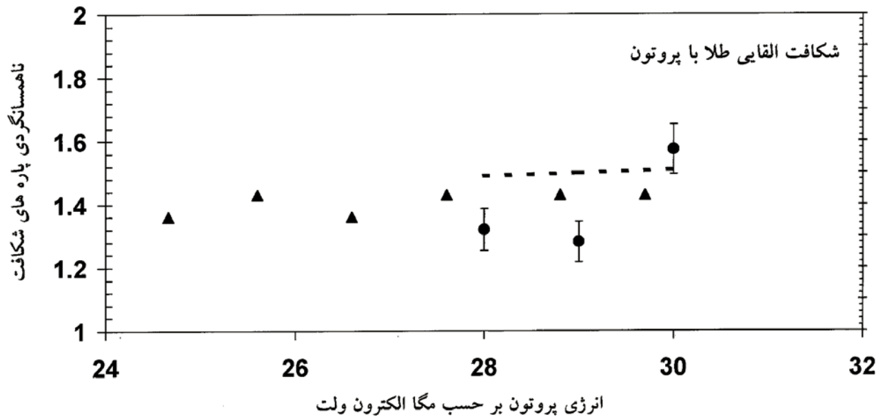
شکل ۱۴. نا همسانگردی زاویه‌ای پاره‌های شکافت عنصر طلا با باریکه پروتون در انرژیهای مختلف. \Delta مربوط به مراجع [۳ و ۴]، منحنی خط چین پیش بینی مدل آماری نقطه زینی استاندارد (بدون در نظر گرفتن اسپین هسته هدف)، و \bullet مربوط به مقادیر اندازه‌گیری شده کنونی است.
