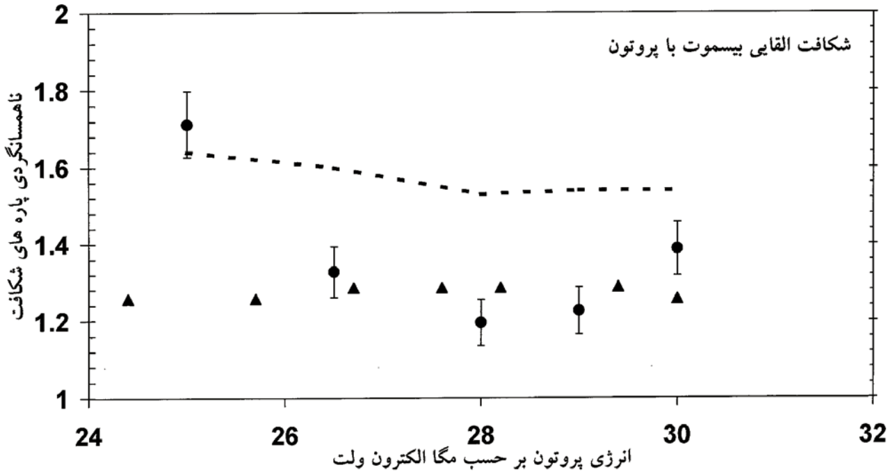
شکل ۱۵. ناهمسانگردی زاویه‌ای پاره‌های شکافت عنصر بیسموت با باریکه پروتون در انرژیهای مختلف. Δ مربوط به مراجع [۴۳]، منحنی خط چین پیش بینی مدل آماری نقطه زینی استاندارد (بدون در نظر گرفتن اسپین هسته هدف)، و ● مربوط به مقادیر اندازه‌گیری شده کنونی است.
