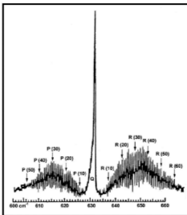
شکل ۱. نمودار طیف دورانی حالت پایه v_3 مولکول CF_4 .
