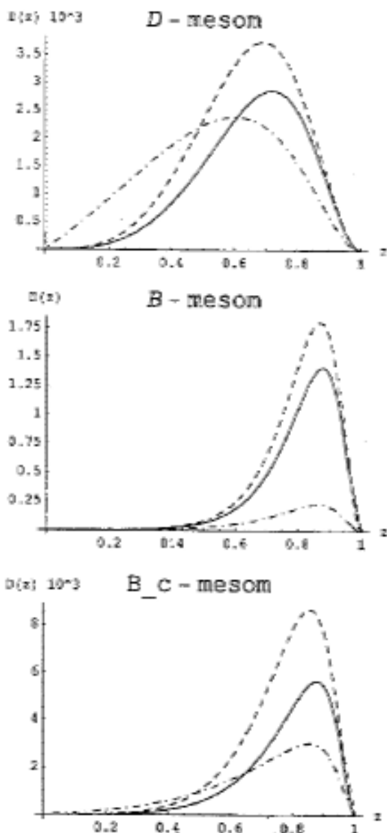
شکل ۲. رفتار توابع ترکش D ۰ (خط پر)، D T (خط چین) و D ave (خط نقطه) در مقیاس ترکش مناسب برای مزونهای D، B و B c
