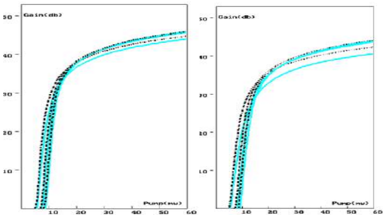
شکل ۹. منحنی بهره تقویت به توان پمپ برای فیبر با پاشندگی انتقال یافته در طول موج پمپ ۰/۹۸ میکرومتر و طولهای بهینه در توانهای پمپ ۱۰، ۲۰ و ۳۰ میلی وات.
