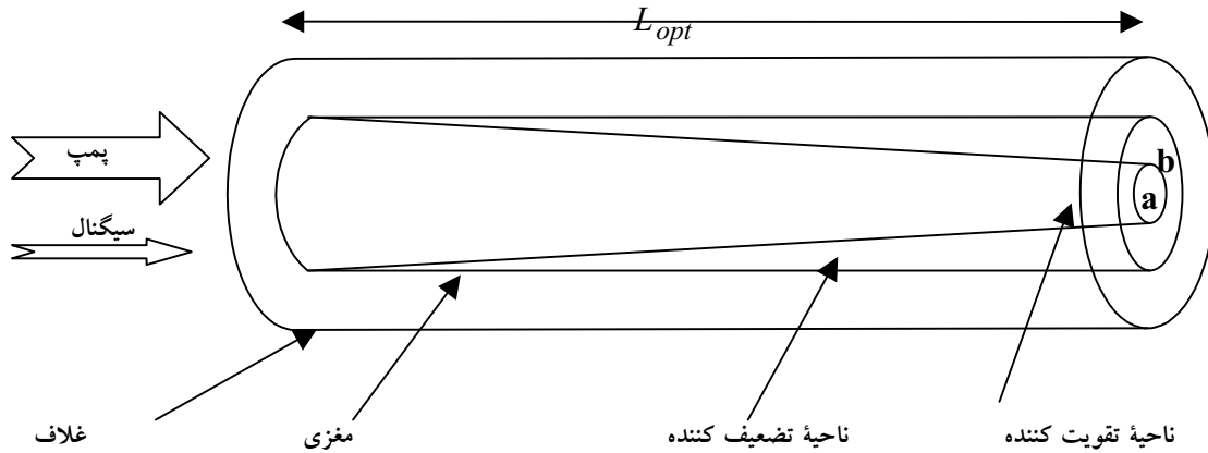
شکل ۱. مناطق تقویت کننده و جذب کننده در مغزی فیبر اریومی که به دلیل شکل توزیع شدت مد اول پمپ به وجود آمده‌اند.
