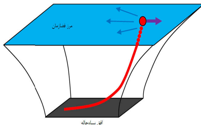
شکل ۱. (رنگی در نسخه الکترونیکی) تصویر ذره متحرک با استفاده از AdS/CFT [۱].
