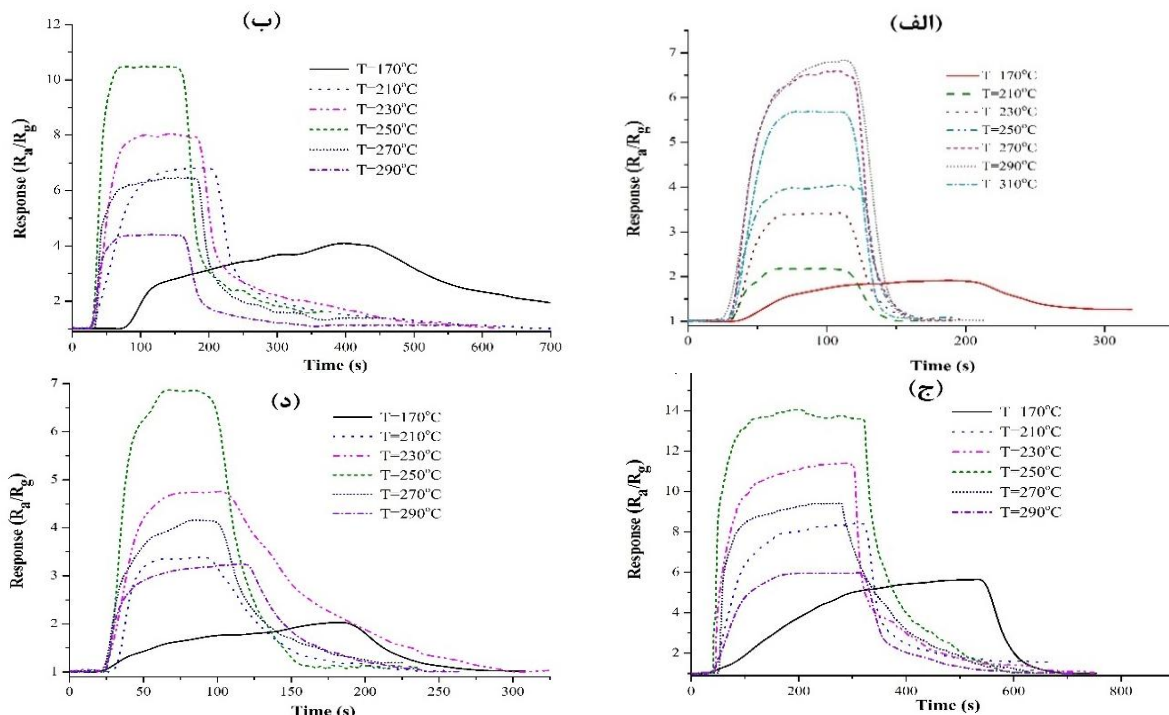
شکل ۵. رنگی در نسخه الکترونیکی) منحنی‌های پاسخ حسگر ساخته شده از نانومیمه‌های کپسول شده ZnO با ناخالصی کروم (الف) ۰.۵٪، (ب) ۰.۵٪، (ج) ۱.۵٪ و (د) ۴.۵٪ به ازای بخار اتانول در دماهای مختلف.
