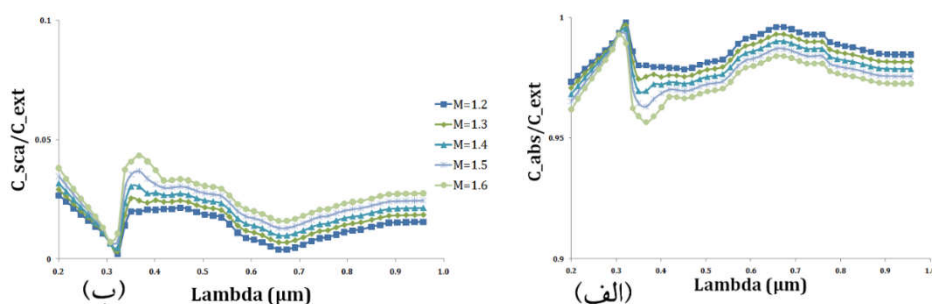
شکل ۵. (رنگی در نسخه الکترونیکی) تغییرات نسبت سطح مقطع های پراکندگی و جذب به سطح مقطع خاموشی بر حسب طول موج نور فرودی وقتی ثابت دی الکتریک محیط متغییر و طول یال نانوذره نقره ثابت (۶۲ نانومتر) باشد.
