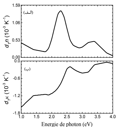
شکل ۲. تغییرات (الف) ضریب شکست و (ب) ضریب خاموشی طلا نسبت به دما بر حسب انرژی فوتون [۷].
