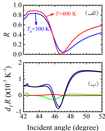
شکل ۳. (رنگی در نسخه الکترونیکی) (الف) ضریب بازتاب حسگر شکل ۱ در دو دمای ۳۰۰ و ۴۰۰ کلونین، (ب) تغییرات گرمایی ضریب بازتاب d_T R (منحنی سیاه) و سهم خواص گرما-نوری فلز طلا (منحنی آبی)، منشور (منحنی سبز) و محیط حسگری (منحنی قرمز) در d_T R .
