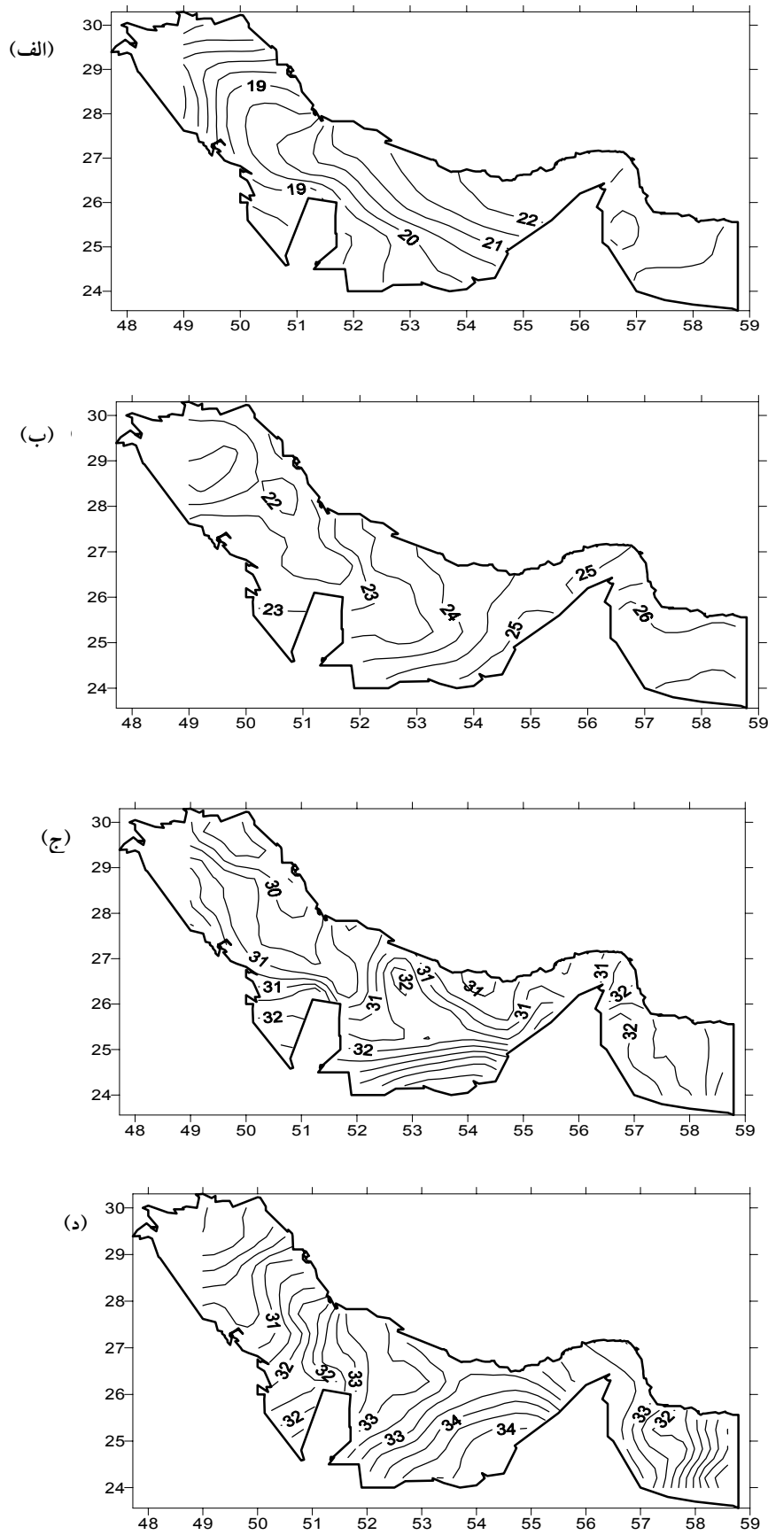
شکل ۳. گردهای فصلی SST در خلیج فارس الف) در فصل زمستان ب) در فصل بهار ج) در فصل تابستان د) در فصل پاییز در سال ۱۹۹۸.
