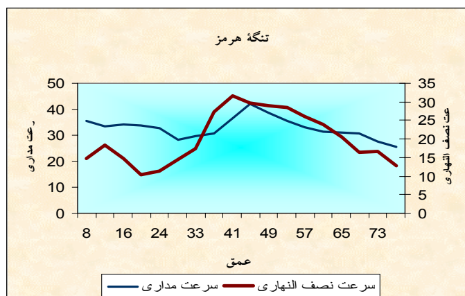
شکل ۲. نیمرخ سرعت جریان آب (cm/s) در راستاهای مداری و نصف النهاری در تنگه هرمز در تاریخ ۱۶ مارس سال ۱۹۹۸ در طول و عرض 06^{\circ}۰۷'۹'' و 26^{\circ}۱۳'۸'' ، در ساعت 05:41 به وقت گرینویچ.
