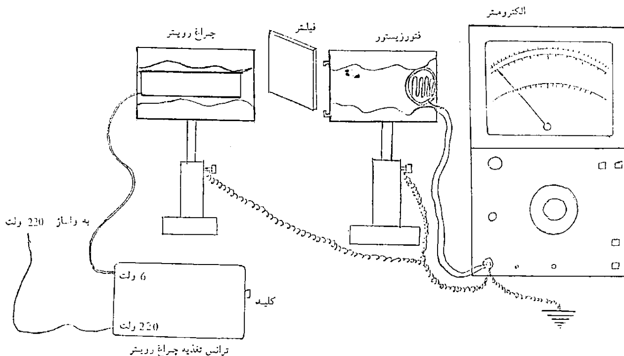
شکل ۲. طرح شماتیک اندازه‌گیری جریان فوتوکاتداکتیو تپته.
