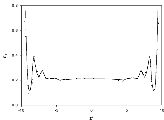
شکل ۸ چگالی بلور مایع با مولکولهای بیضی وار موازی دیوارهها برحسب فاصله کاهش یافته، برای کسر پکیدگی 0/5 و نسبت قطر بزرگ به قطر کوچک 5 خط ممتد مربوط به محاسبت این مقاله و نقاط مربوط به نتایج شبیه سازی مونت-کارلو می باشند.
