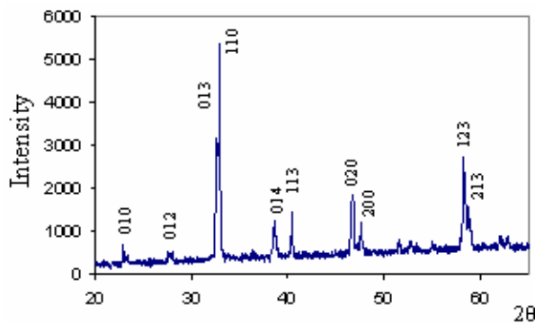
شکل ۴. الگوی پراش پودری نمونه YBCO بدون نقره.
