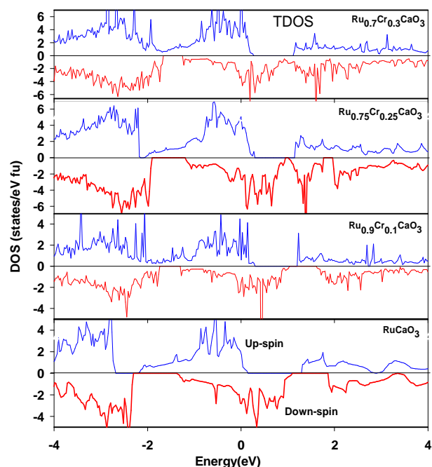
شکل ۲. چگالی حالات کل و برآورد انرژی شکافتگی تبدلی برای Ru_{1-x}Cr_xCaO_3 .
