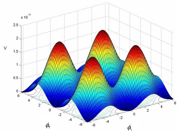
شکل ۴. منحنی پتانسیل بر حسب \phi_1 و \phi_2 .
