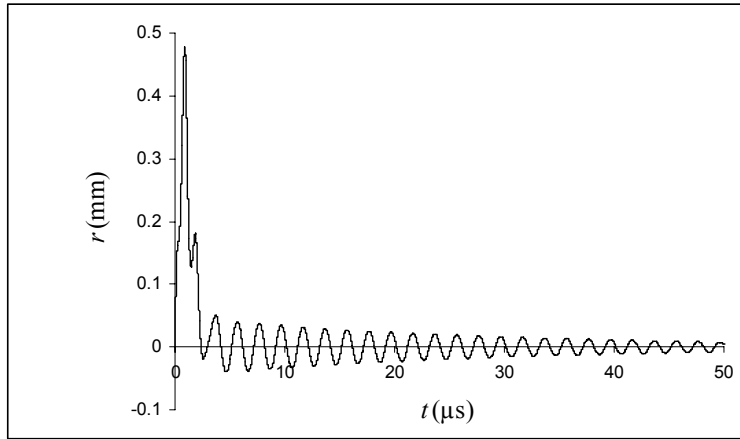
شکل ۵. منحنی موقعیت r بر حسب زمان در حالت \kappa=1 برای H^+ . V_{ac}=54\text{ V} , V_{dc}=0\text{ V} , f=1\text{ MHz} . r_0=15\text{ mm} متناظر با a_z=0 و q_z=2/35 گیراندازی صورت می گیرد.
