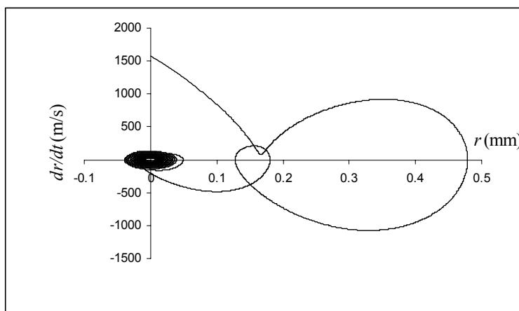
شکل ۷. منحنی فضای فاز r-dr/dt برای H^+ در حالت \kappa=1 . V_{ac}=54\text{ V} , V_{dc}=0\text{ V} , f=1\text{ MHz} . r_0=15\text{ mm} متناظر با a_z=0 و q_z=2/35 گیراندازی صورت می گیرد.
