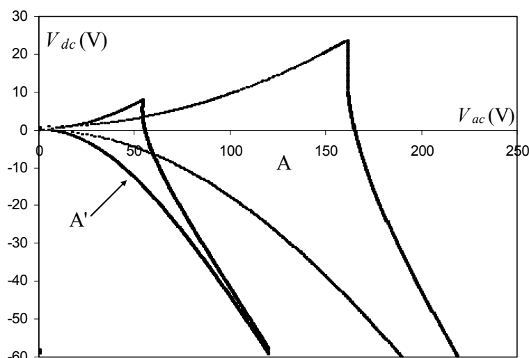
شکل ۹. نمودار ولتاژ مستقیم نسبت به ولتاژ متناوب در حالت \kappa=1 متناظر با f=1\text{ MHz} و r_0=15\text{ mm} . ناحیه A' برای H^+ و ناحیه A برای H^+ رسم شده است.
