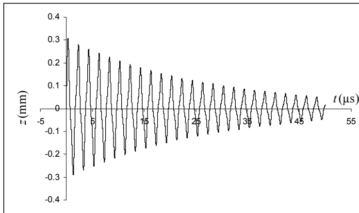
شکل ۶. منحنی موقعیت z بر حسب زمان در حالت \kappa=1 برای H^+ . V_{ac}=54\text{ V} , V_{dc}=0\text{ V} , f=1\text{ MHz} . r_0=15\text{ mm} متناظر با a_z=0 و q_z=2/35 گیراندازی صورت می گیرد.
