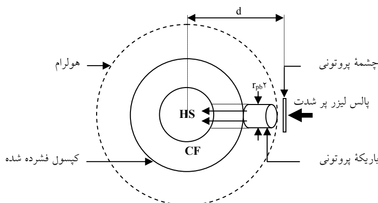
شکل ۱. نمایش طرح وار ایده اشتعال سریع با هدف کروی. HS و CF روی شکل به ترتیب بیانگر سوخت سرد و ناحیه داغ اشتعالی می باشند.
