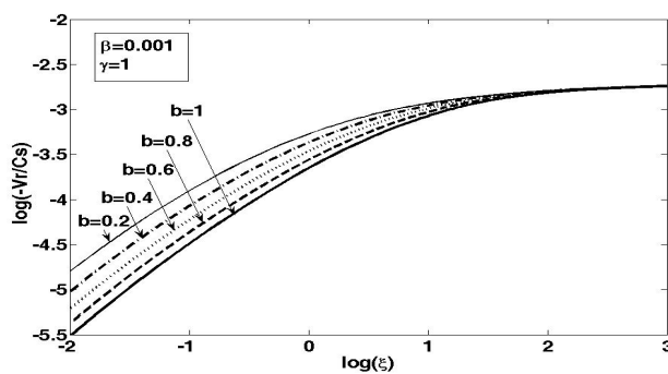
شکل ۱. مولفه شعاعی سرعت که تابعی از فاصله است. با ثابت بودن مقادیر q=0.003 ، \beta=0.001 ، \gamma=1 با تغییر اثر میدان مغناطیسی به ازای مقادیر b=0.2 ، b=0.4 ، b=0.6 ، b=0.8 ، b=1 نمودار رسم شده است.
