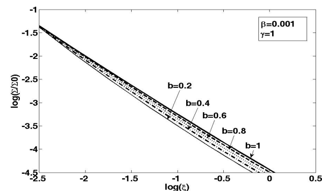
شکل ۳. نمودار چگالی سطحی که تابعی از فاصله است. با ثابت بودن مقادیر q=0.003 ، \beta=0.001 ، \gamma=1 با تغییر میدان مغناطیسی به ازای b=0.2 ، b=0.4 ، b=0.6 ، b=0.8 ، b=1 نمودار رسم شده است.
