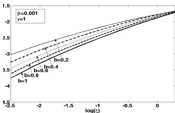
شکل ۴. نمودار آهنگ برافزایش جرم که تابعی از فاصله است. با ثابت بودن مقادیر q=0.003 ، \beta=0.001 ، \gamma=1 با تغییر میدان مغناطیسی به ازای b=0.2 ، b=0.4 ، b=0.6 ، b=0.8 ، b=1 نمودار رسم شده است.
