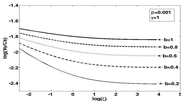
شکل ۲. نمودار مولفه سمتی سرعت که تابعی از فاصله است. با ثابت بودن مقادیر q=0.003 ، \beta=0.001 ، \gamma=1 با تغییر میدان مغناطیسی به ازای b=0.2 ، b=0.4 ، b=0.6 ، b=0.8 ، b=1 نمودار رسم شده است.
