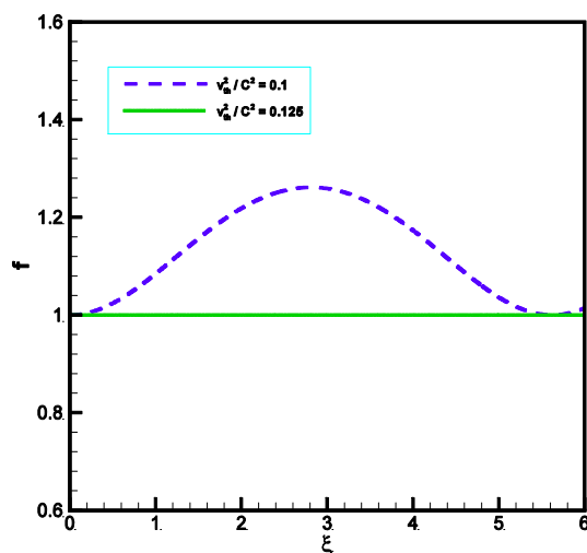
شکل ۲. تغییر پهنای لیزر برای \eta = 0 با \alpha_{NL} = 4 .
