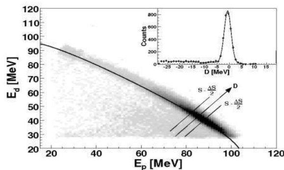
شکل ۷. سینماتیک کانال تجزیه سه جسمی برای واکنش پراکنندگی دوترون-دوترون با استفاده از دو متغیر S و D [۷].
