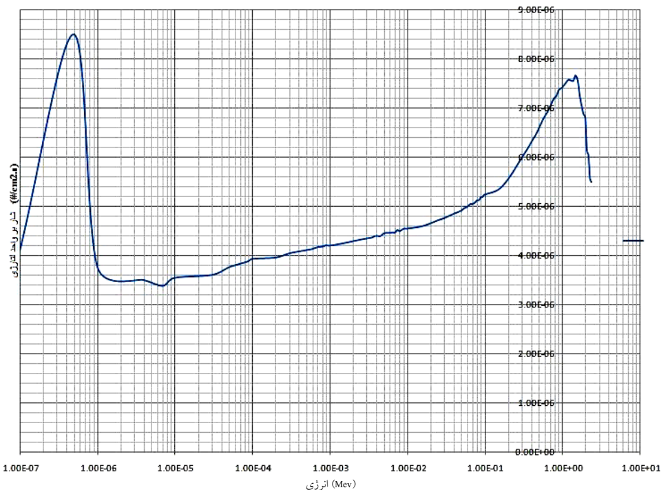
شکل ۴. توزیع انرژی شار نوترونی بر واحد لتارژی.
