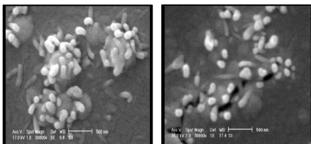
شکل ۳. تصاویر SEM، با بزرگنمایی 500\times نانومتر مربوط به لایه نازک \text{TiO}_2\text{-SnO}_2 با زیرلایه شیشه و آلومینیوم/شیشه، تحت دمای بازپخت 550^\circ\text{C} درجه سانتی گراد.
