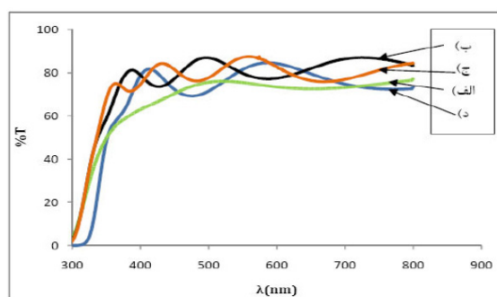
شکل ۱۰. طیف عبوری لایه‌های نازک \text{TiO}_2\text{-SnO}_2 با زیرلایه شیشه تحت دمای بازپخت: (الف) 550^\circ\text{C} درجه سانتی‌گراد، (ب) 500^\circ\text{C} درجه سانتی‌گراد، (ج) 450^\circ\text{C} درجه سانتی‌گراد و (د) لایه نازک \text{TiO}_2 .
