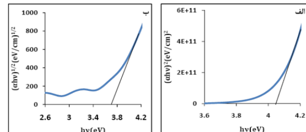
شکل ۱۳. گاف انرژی لایه نازک TiO-SnO برای گذار مجاز دمای بازپخت ۴۵۰ درجه سانتی گراد (الف) مستقیم، (ب) غیرمستقیم.
