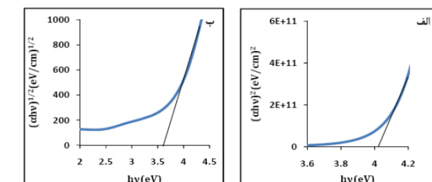
شکل ۱۱. گاف انرژی لایه نازک TiO-SnO برای گذار مجاز دمای بازپخت ۵۵۰ درجه سانتی گراد: (الف) مستقیم، (ب) غیرمستقیم.
