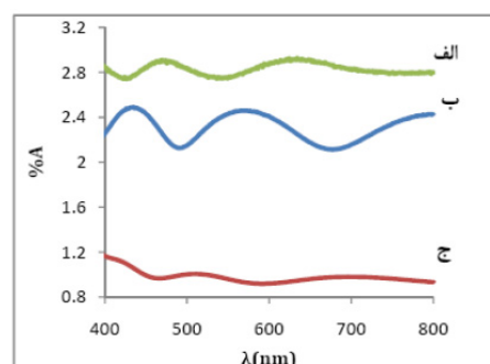
شکل ۹. طیف جذبی لایه‌های نازک \text{TiO}_2\text{-SnO}_2 با زیرلایه آلومینیوم تحت دمای بازپخت (الف) 550^\circ\text{C} درجه سانتی‌گراد، (ب) 500^\circ\text{C} درجه سانتی‌گراد، (ج) 450^\circ\text{C} درجه سانتی‌گراد.
