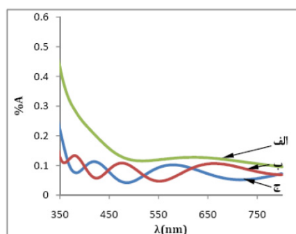
شکل ۸. طیف جذبی لایه‌های نازک \text{TiO}_2\text{-SnO}_2 با زیرلایه شیشه تحت دمای بازپخت: (الف) 550^\circ\text{C} درجه سانتی‌گراد، (ب) 500^\circ\text{C} درجه سانتی‌گراد، (ج) 450^\circ\text{C} درجه سانتی‌گراد.
