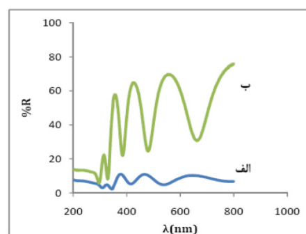
شکل ۹. طیف بازتابی لایه نازک \text{TiO}_2\text{-SnO}_2 با زیرلایه (الف) شیشه، (ب) آلومینیوم، تحت دمای بازپخت 550^\circ\text{C} درجه سانتی‌گراد.
