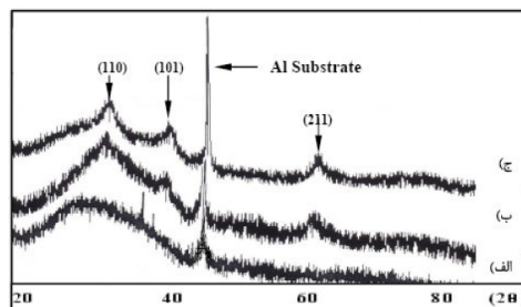
شکل ۲. آنالیز پراش پرتوی ایکس لایه نازک \text{TiO}_2\text{-SnO}_2 با زیرلایه آلومینیوم/شیشه تحت دمای بازپخت: (الف) 450^\circ\text{C} درجه سانتی گراد، (ب) 500^\circ\text{C} درجه سانتی گراد، (ج) 550^\circ\text{C} درجه سانتی گراد.
