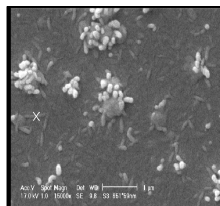
شکل ۴. تصویر SEM، با بزرگنمایی 1\times میکرومتر مربوط به لایه نازک \text{TiO}_2\text{-SnO}_2 با زیرلایه آلومینیوم/شیشه، تحت دمای بازپخت 550^\circ\text{C} درجه سانتی گراد.
