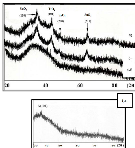
شکل ۱. آنالیز پراش پرتو ایکس لایه نازک TiO - SnO با زیرلایه شیشه، تحت دمای بازپخت: الف) ۴۵۰ درجه سانتی‌گراد، ب) ۵۰۰ درجه سانتی‌گراد، ج) ۵۵۰ درجه سانتی‌گراد، د) آنالیز پراش پرتو ایکس لایه نازک TiO با زیر لایه شیشه تحت دمای بازپخت ۵۰۰ درجه سانتی‌گراد.
