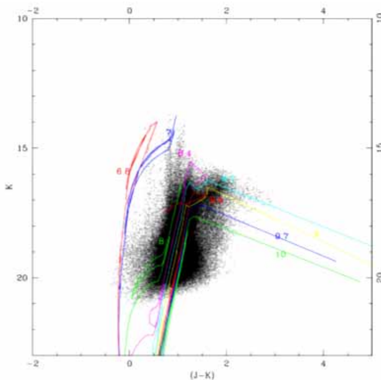
شکل ۱۹. (رنگی در نسخه الکترونیکی) نمودار قدر رنگ کهکشان M33 با خطوط هم سن.
