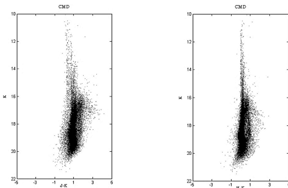
شکل ۱۴. نمودار قدر رنگ برای کهکشان M33 پس از بررسی ۸۰۱ فهرست ستاره‌ای حاصل از تصویربرداری توسط دوربین WFCAM.
