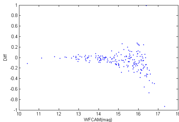
شکل ۵. توزیع قدر- اختلاف قدر حاصل از مقایسه دو فهرست ستاره‌ای ۲MASS و WFCAM.
