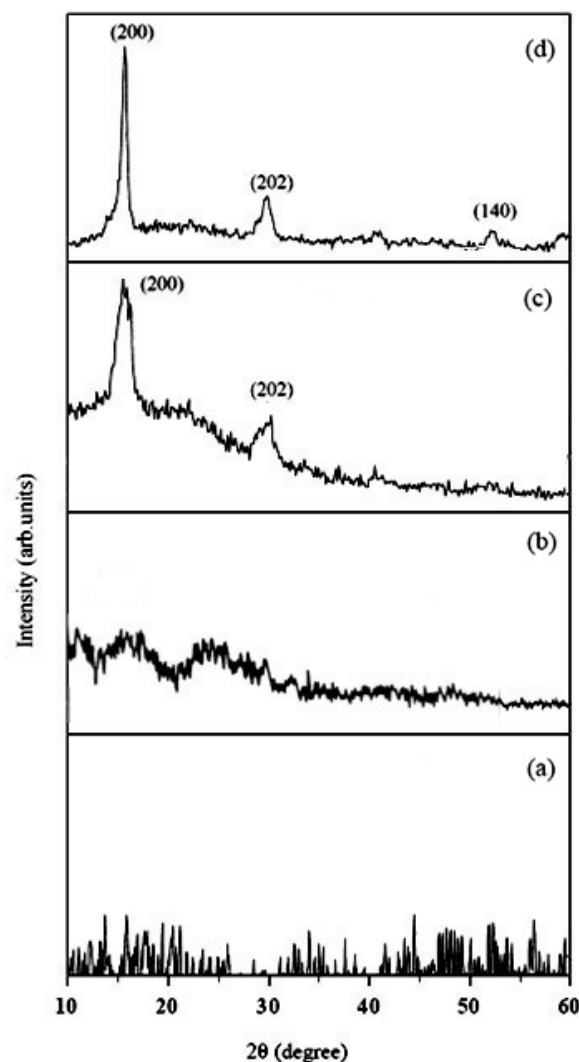
شکل ۱۳. طرح پراش اشعه X لایه WO_3 (a) 25^\circ C ، (b) 120^\circ C ، (c) 300^\circ C ، (d) 500^\circ C .
