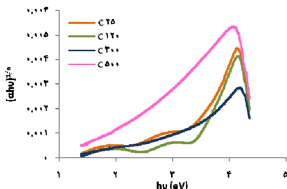
شکل ۷. (رنگی در نسخه الکترونیکی) نمودار (\alpha h\nu)^{1/n} برحسب انرژی لایه V_2O_5 در ضخامت ۲۰۰ nm در دماهای بازپخت متفاوت.
