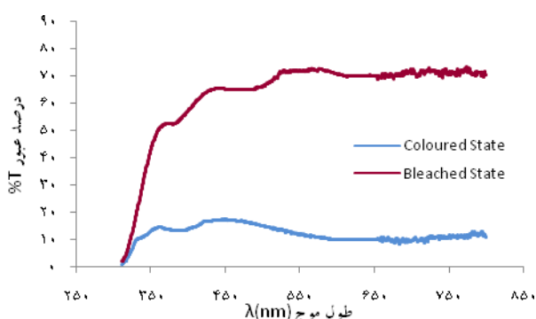
شکل ۱۹. (رنگی در نسخه الکترونیکی) اثر الکتروکرومیک با اعمال ولتاژ +۱/۵ تا -۱/۵ ولت.
