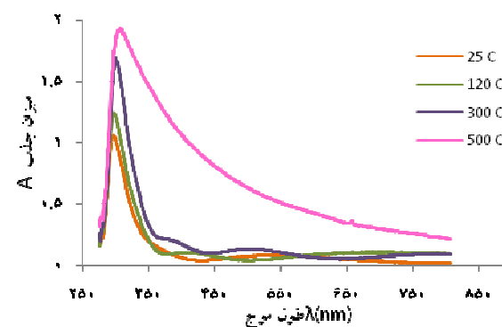
شکل ۶. (رنگی در نسخه الکترونیکی) میزان جذب اپتیکی لایه WO_3 برحسب طول موج در ضخامت ۲۰۰ nm در دماهای بازپخت متفاوت.
