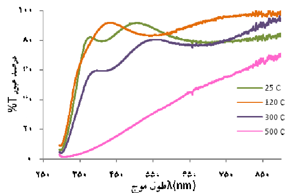
شکل ۴. (رنگی در نسخه الکترونیکی) درصد عبور اپتیکی لایه WO_3 برحسب طول موج در ضخامت ۲۰۰ nm در دماهای بازپخت متفاوت.
