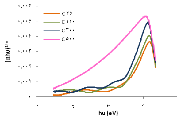
شکل ۸. (رنگی در نسخه الکترونیکی) نمودار (\alpha h\nu)^{1/n} برحسب انرژی لایه WO_3 در ضخامت ۲۰۰ nm در دماهای بازپخت متفاوت.
