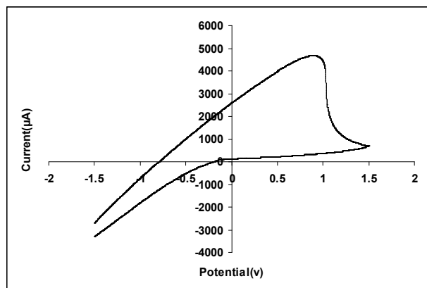
شکل ۱۷. چرخه ولتامتری لایه اکتروکرومیک \text{SnO}_2\text{:F} - \text{WO}_3 در محلول \text{HClO}_4 .
