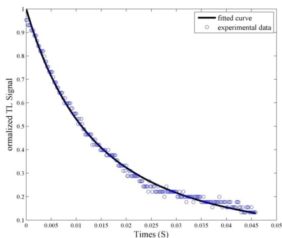
شکل ۵. مقایسه تغییرات نسبی سیگنال TL اندازه‌گیری شده برحسب زمان با محاسبات نظری در نمونه S ۲ .
