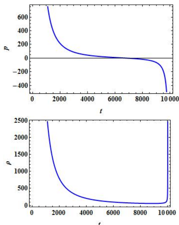
شکل ۴. فشار (بالا) و چگالی انرژی (پایین) در تکنیکی نوع سوم به ازای n = 0.5 و q = 0.5 .
