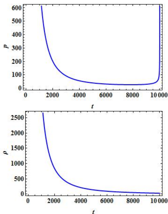
شکل ۳. فشار و چگالی انرژی در تکنیکی نوع دوم به ازای n=1/5 و q=0/5 .
