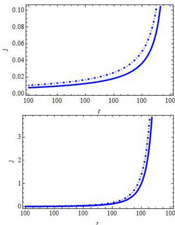
شکل ۵. نمودار J بر حسب زمان به ازای b = \frac{1}{5} (خط نقطه چین) و b = \frac{7}{10} (خط ممتد)، در نزدیکی تکنیکی نوع دوم (شکل بالایی)، و در نزدیکی تکنیکی نوع سوم (شکل پایینی). قانون دوم ترمودینامیک در نزدیکی تکنیکی نوع دوم و سوم برقرار است.
