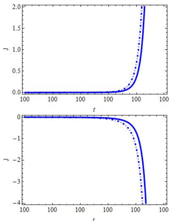
شکل ۲. نمودار J بر حسب زمان به ازای b = \frac{1}{5} (خط نقطه‌چین) و b = \frac{7}{10} (خط ممتد) و t_s = 100 ، n = 2 و P(99/999) = 0.1 (شکل پایینی) و \dot{P}(99/999) = 0.1 (شکل بالایی). برقراری قانون دوم ترمودینامیک در نزدیکی شکافتگی بزرگ وابسته به شرایط اولیه‌ای است که در نظر گرفته می‌شود. در شکل‌های بالا شرایط اولیه یکسان است، اما تغییر در مقدار n نتیجه را تغییر داده است.
