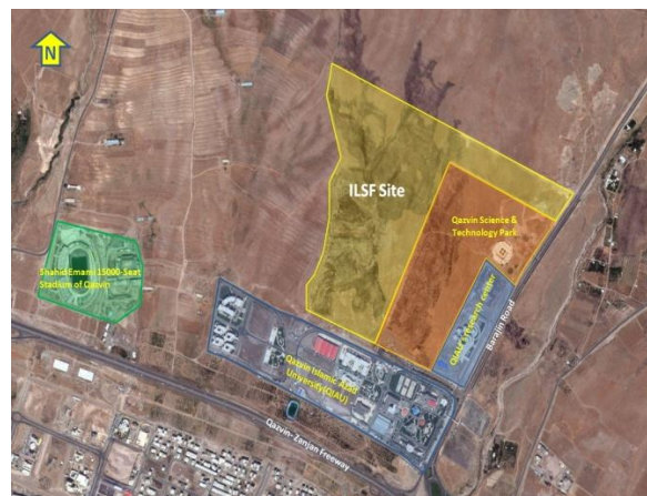
شکل ۱۳. تصویر هوایی از محل ساختگاه طرح چشمه نور ایران همراه با جانمایی ساختمان‌ها در آن (راست) و نتایج مطالعات لرزه نگاری (چپ).
