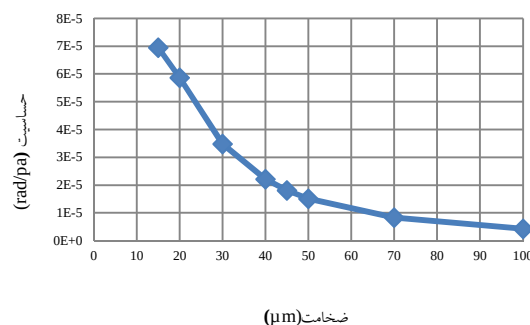
شکل ۵. تغییر حساسیت حسگر با تغییرات ضخامت دریاچه.
