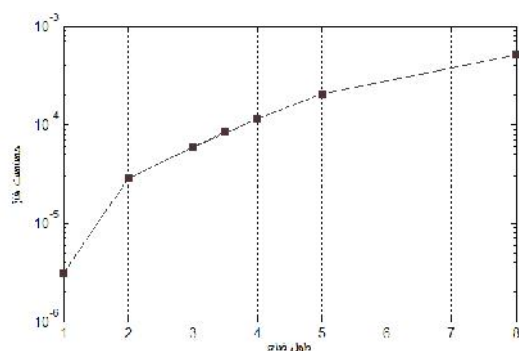
شکل ۶. تغییر حساسیت حسگر با تغییرات ضلع دریاچه مربعی.
