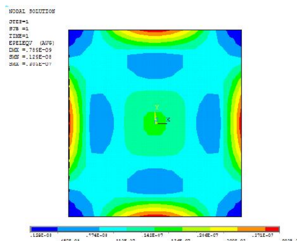
شکل ۴. (رنگی در نسخه الکترونیکی) کرنش فون میزس دریچه مربعی به ضلع ۳ mm وضخامت ۲۰ μm با اعمال فشار یکنواخت یک پاسکال.
