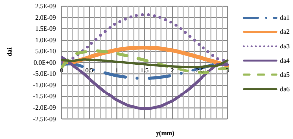
شکل ۴. (رنگی در نسخه الکترونیکی) تغییرات ضرایب بیضوی ضریب شکست ( da_i ) موج‌بر تحت اعمال فشار یکنواخت یک پاسکال در عمق ۵ میکرومتری موج‌بر.
