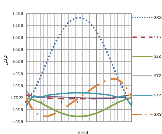
شکل ۳. (رنگی در نسخه الکترونیکی) کرنش در عمق ۵ میکرومتری در محل موج بر (با فاصله ۱۰۰ میکرومتر از لبه دریچه) بر اثر اعمال فشار یکنواخت یک پاسکال.
