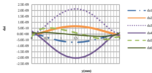
شکل ۴. (رنگی در نسخه الکترونیکی) تغییرات ضرایب بیضوی ضریب شکست ( da_i ) موج‌بر تحت اعمال فشار یکنواخت یک پاسکال در عمق ۵ میکرومتری موج‌بر.
